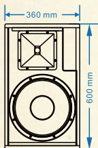
主视图
